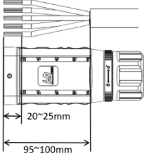
صورة رقم 10: تحضير الكابل
