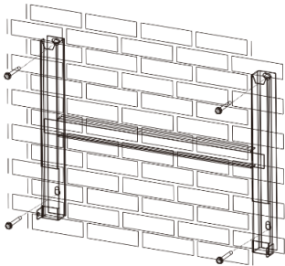
איור 5: התקנת מתלה קיר
