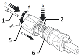
Sl. 14: Umetanje žica
