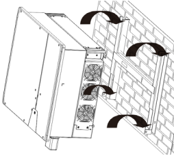
Fig. 6: Engatar o inversor no suporte de parede
