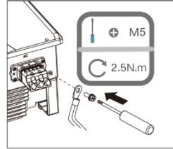
17. att. Zemējuma pieslēgšana
