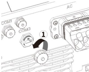
18 pav. Nuimkite gaubtelį
