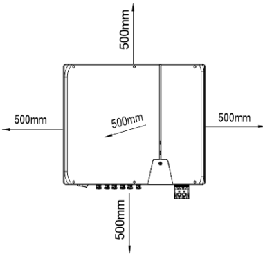
Fig. 3.1: Dispositivo na instalação exterior
