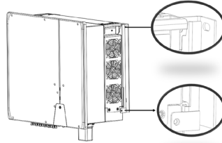
Fig. 7: Kontrollera att enheten sitter ordentligt
