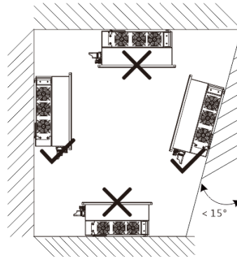
Obr. 2: Povolená poloha pro instalaci
