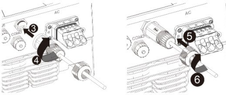
Şek. 22: Ağ kablosunun bağlanması
