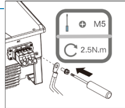
Rys. 17: Podłączenie uziemienia
