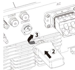
Fig. 19: Conectar o adaptador Wi-Fi
