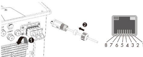
Rys. 20: Wprowadzanie kabla sieciowego
