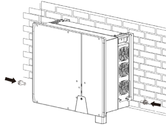
איור 8.1: הידוק הממיר
