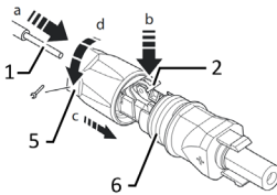
Imm. 14: Introdurre i fili
