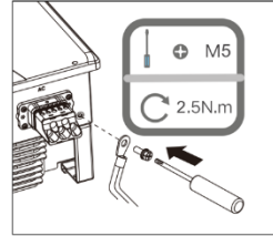
Fig. 17: Tilkobling av jording
