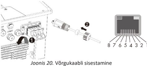
Joonis 20. Võrgukaabli sisestamine
