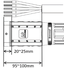
Imm. 10: Preparare il cavo
