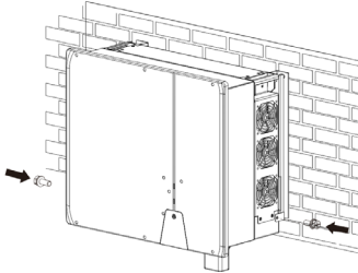
Joonis 8.1. Inverteri kinnitamine
