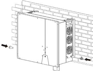
Fig. 8.1: Fixarea redresorului
