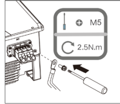
17 pav. Prijunkite įžeminimą
