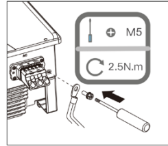
Фиг. 17: Свързване на заземяването
