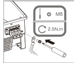
Εικ. 17: Σύνδεση γείωσης
