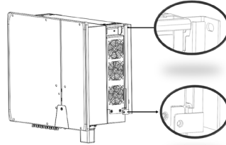
7. att. Ierīces fiksācijas pārbaude
