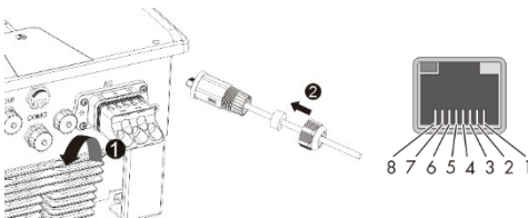
Afb. 20: Netwerkkabel invoeren
