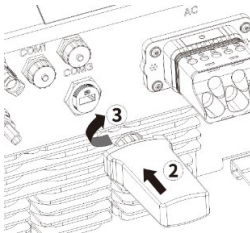
איור 19: חיבור בונן WLAN
