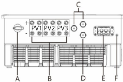
8.2 pav. Prijungimo pusė. Eksplikacija
