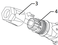
Abb. 15: Einsatz in Hülse schieben
