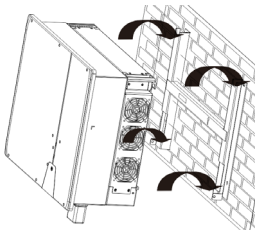
Фиг. 6: Окачване на инвертора към стенния носач
