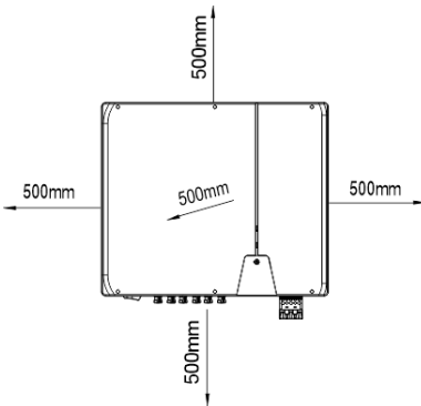
3.1. att. Ārpus telpām uzstādīta ierīce
