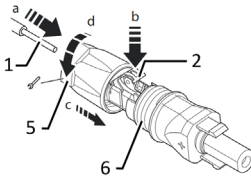
Фиг. 14: Вкарване на проводници
