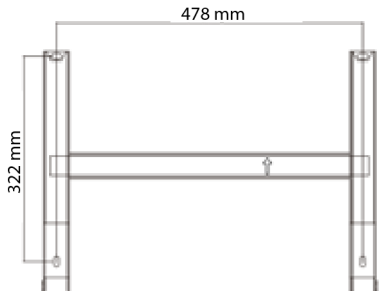
איור 4: קידוחים להתקנה על הקיר
