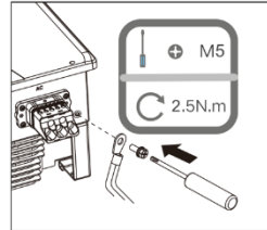
Sl. 17: Priklpite ozemljitev
