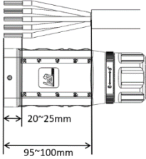
איור 10: הכנת הכבל
