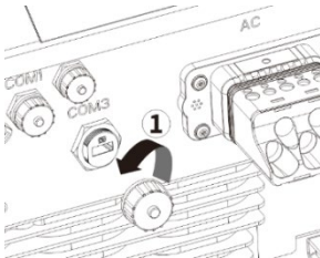
Rys. 18: Zdejmowanie pokrywki
