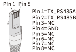
Fig. 21: Distribución de conexiones de cables
