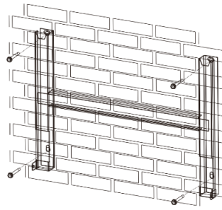
Fig. 5: Montaje del soporte mural
