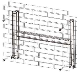
Fig. 5 : Montage du support mural
