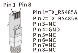
Fig. 21: Alocarea racordului cablului
