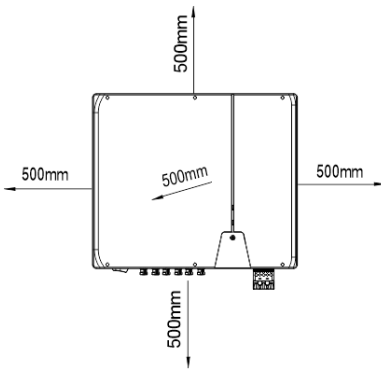
Kuva 3.1: Laitte ulkoasennuksessa
