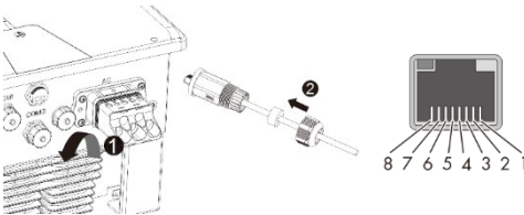
Fig. 20: Føre inn nettverkskabel
