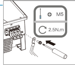
Fig. 17: Estabelecer a ligação à terra
