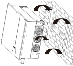
Afb. 6: Omvormer in de wandhouder hangen
