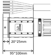
Abb. 10: Kabel vorbereiten
