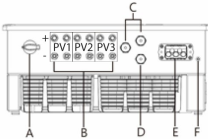
Şek. 8.2: Bağlantı tarafı: Açıklamalar
