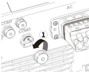
Sl. 18: Uklanjanje pokrova
