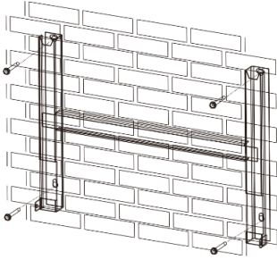
صورة رقم 5: التركيب على الحامل الجداري
