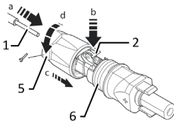
14. ábra: Az erek bevezetése
