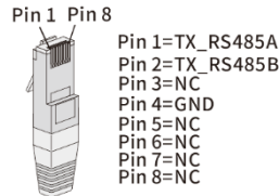
Joonis 21. Kaabli ühendamise paigutus
