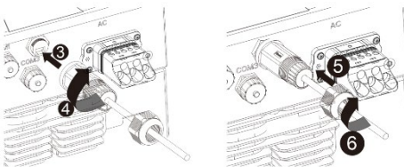
Rys. 22: Podłączanie kabla sieciowego
