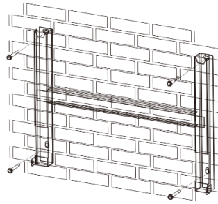
Afb. 5: Montage van de wandhouder
