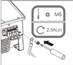
איור 17: חיבור הארקה
