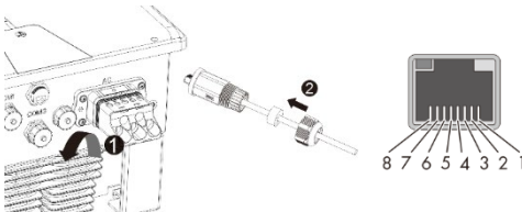
Obr. 20: Zasunutí síťového kabelu
