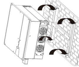
صورة رقم 6: قم بتعليق العاكس في الحامل الجداري
