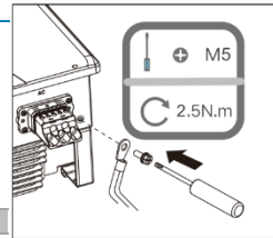
Afb. 17: Aarding aansluiten
