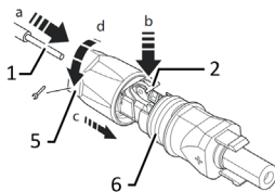
Fig. 14: Insert wires
