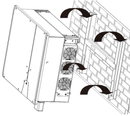
Fig. 6: Acroșarea redresorului în suportul de perete
