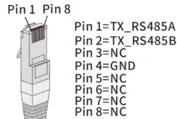
Imm. 21: Assegnazione dei collegamenti dei cavi
