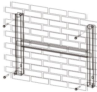
Фиг. 5: Монтаж на стенния носач
