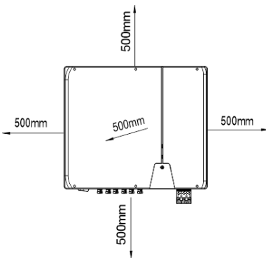
Afb. 3.1: Apparaat bij buiteninstallatie
