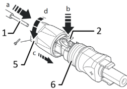
Joonis 14. Soonte sisestamine
