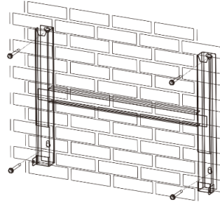
Şek. 5: Duvar tutucusunun montajı
