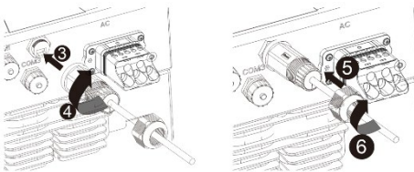
Fig. 22: Racordarea cablului de rețea
