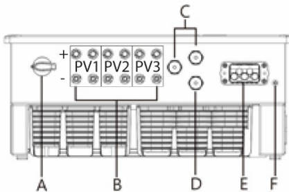
Fig. 8.2 : Côté branchement : Légende
