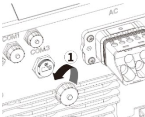
Abb. 18: Abdeckung entfernen
