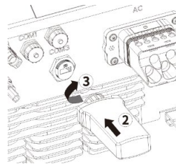
Sl. 19: Priključivanje WiFi štapića
