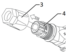
Fig. 15: Introduzir o inserto no casquilho
