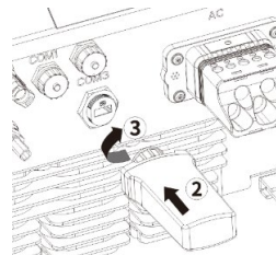
Abb. 19: WLAN-Stick anschließen
