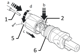
صورة رقم 14: أدخل الأسلاك
