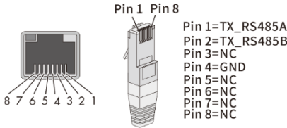
איור 21:22 הקצאת חיבורי הכבל
