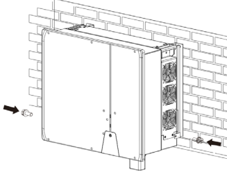
Şek. 8.1: İnverterin sabitlenmesi
