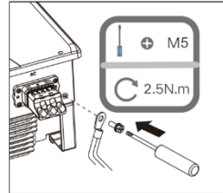
Sl. 17: Priključivanje uzemljenja
