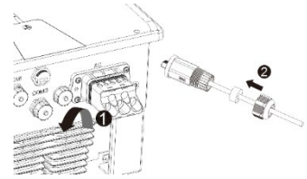
איור 20: השחלת כבל רשת
