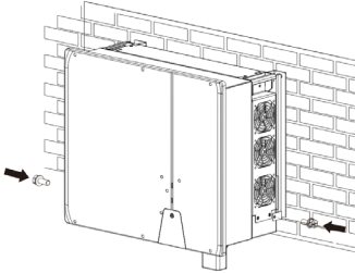
Imm. 8.1: Fissare l'inverter
