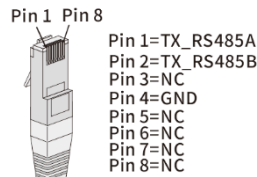
Fig. 21: Ledningsføring
