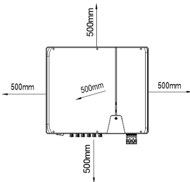
Joonis 3.1. Seade välja paigaldamisel
