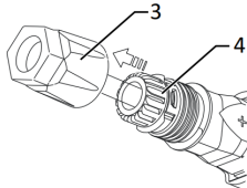
Fig. 15: Skjuta in insatsen i hylsan
