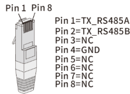
Obr. 21: Osazení kabelové přípojky
