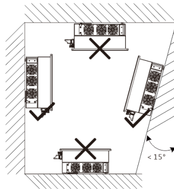
Joonis 2. Lubatud paigaldusasend
