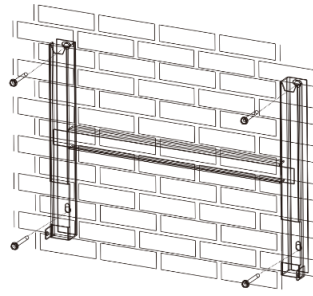
Εικ. 5: Συναρμολόγηση στηρίγματος τοίχου
