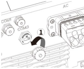
Şek. 18: Kapağı çıkarma
