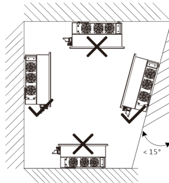
Fig. 2: Tillatt oppstillingsposisjon
