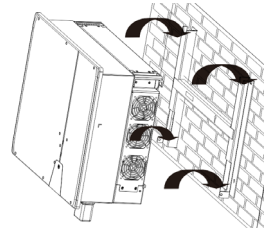
איור 6: תליית הממיר על מתלה הקיר
