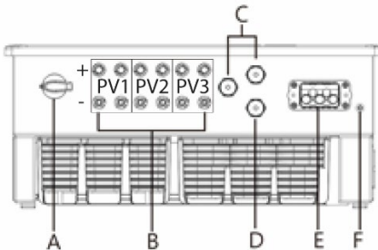
8.2. att. Pieslēguma puse: Apraksts
