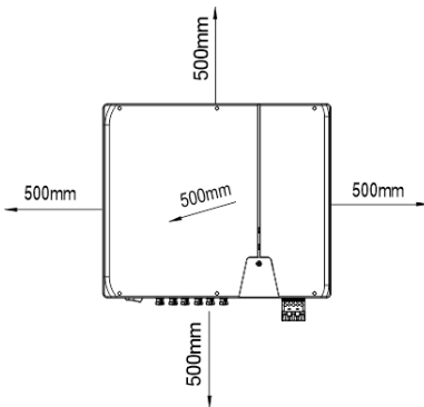
Фиг. 3.1: Уред при инсталиране на открито
