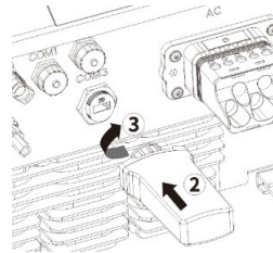
19 pav. Prijunkite WLAN modulį
