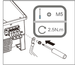
Fig. 17 : Raccordement de la terre
