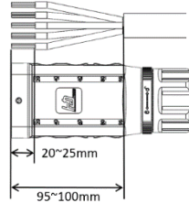
Fig. 10 : Préparer le câble
