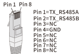
Фиг. 21: Заемане на свързването на кабела
