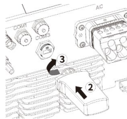
Fig. 19: Tilslut WLAN-stik
