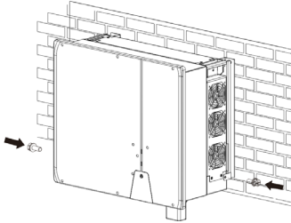
Εικ. 8.1: Στερέωση μετατροπέα
