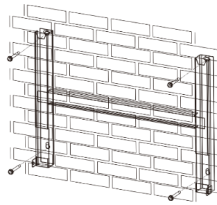
Fig. 5: Montering af vægholderen
