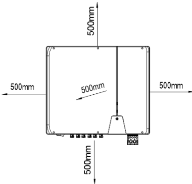
Fig. 3.1: Aparat la instalarea la exterior
