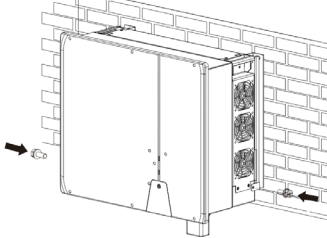
8.1 pav. Pritvirtinkite inverterį
