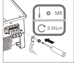
Şek. 17: Topraklamanın bağlanması
