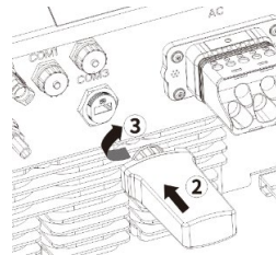
Fig. 19: Ansluta WLAN-stickan
