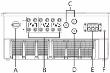
Kuva 8.2: Liitäntäpuoli: Kuvateksti
