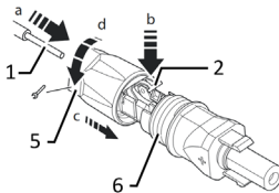
Sl. 14: Vpeljite žile
