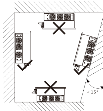
Εικ. 2: Επιτρεπόμενη θέση τοποθέτησης
