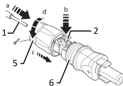
Afb. 14: Draden invoeren
