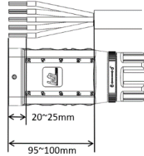
Sl. 10: Priprema kabela
