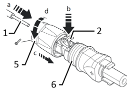
Obr. 14: Zavedenie žíl
