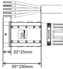
Rys. 10: Przygotowanie kabla
