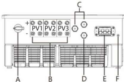
8.2. ábra: Csatlakozási oldal: Jelmagyarázat
