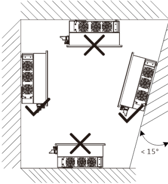
صورة رقم 2: موقع التركيب المسموح به
