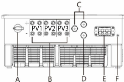
Sl. 8.2: Priključna strana: Legenda
