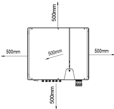
Sl. 3.1: Naprava pri namestitvi na prostem
