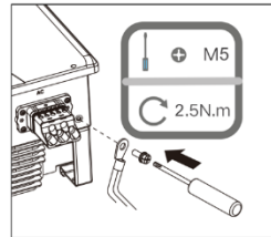
Fig. 17: Tilslut jordforbindelsen
