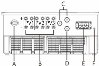
Imm. 8.2: Lato di collegamento: Legenda
