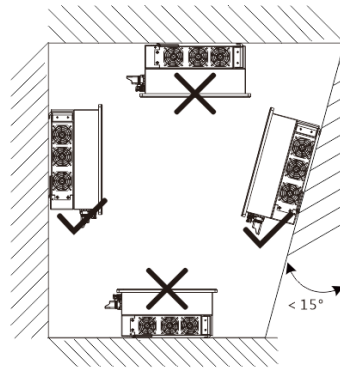
Fig. 2: Posição de instalação permitida
