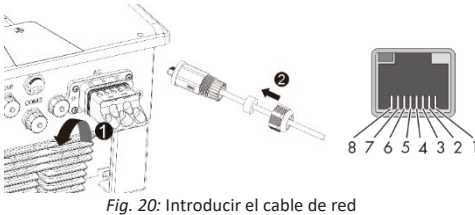
Fig. 20: Introducir el cable de red
