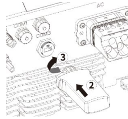
Şek. 19: WLAN-Stick'in bağlanması
