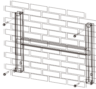
Kuva 5: Seinäkiinnikkeen asennus
