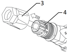
15. att. Ieliktna ievietošana čaulā
