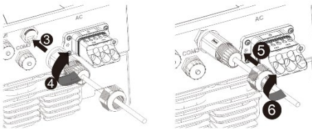
Imm. 22: Collegare il cavo di rete
