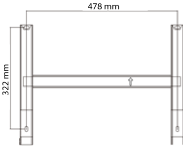
Εικ. 4: Οπές για επιτοίχια τοποθέτηση
