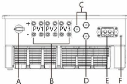
Fig. 8.2: Lado de conexión: Leyenda
