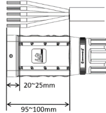
Fig. 10: Klargjøring av kabelen
