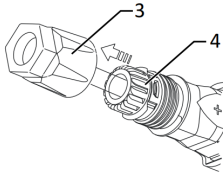
Kuva 15: Työnnä sisus holkkiin
