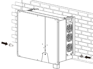
Fig. 8.1: Fastgørelse af vekselretter
