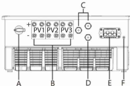
Joonis 8.2. Ühenduspool: Legend
