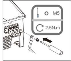
Obr. 17: Pripojenie uzemnenia
