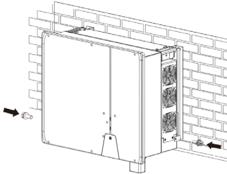
Obr. 8.1: Upevnenie striedača
