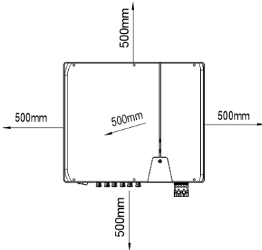
3.1. ábra: Készülék felszerelése kültéren
