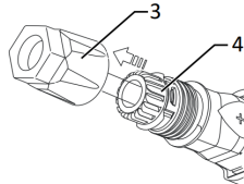
איור 15: דחף את חומר ההידוק לתוך קסווה
