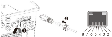
Kuva 20: Aseta verkkojohto paikalleen
