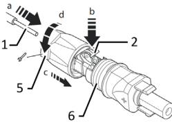
Rys. 14: Wprowadzić żyły
