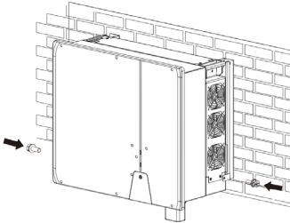
8.1. att. Invertora nostiprināšana
