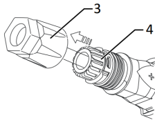
Фиг. 15: Плъзгане на вложката във втулката
