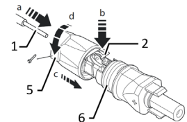
איור 14: השחלת חוטים
