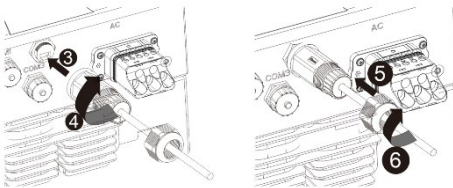
Фиг. 22: Свързване на мрежов кабел
