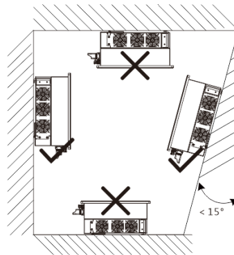
Afb. 2: Toegestane opstelstand
