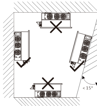
Sl. 2: Dopušten položaj postavljanja
