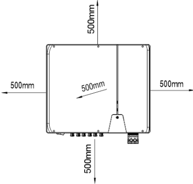
Şek. 3.1: Açık alanlara kurulumda cihaz
