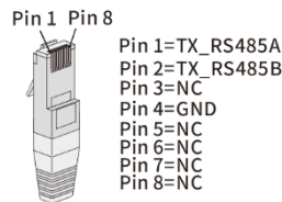
Afb. 21: Indeling kabelaansluiting
