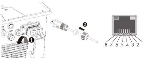
Sl. 20: Vpeljite omrežni kabel
