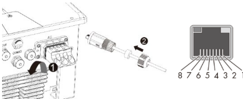
Sl. 20: Uvođenje mrežnog kabela
