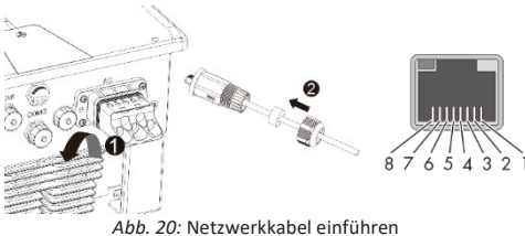
Abb. 20: Netzwerkkabel einföhren
