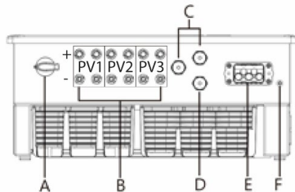
איור 8.2: צד החיבור: מקרא
