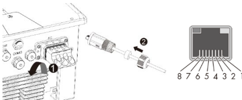
Obr. 20: Zavedenie sieťového kábla
