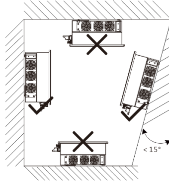
Şek. 2: İzin verilen kurulum yeri
