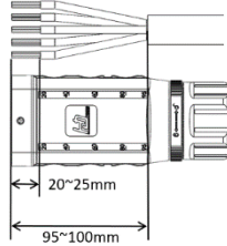
Kuva 10: Kaapelin valmistelu
