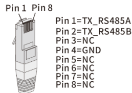
Obr. 21: Obsadenie káblvej prípojky
