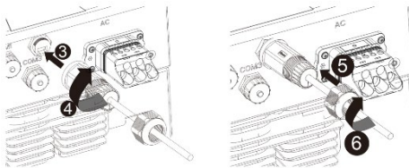
Sl. 22: priklop omrežnega kabla
