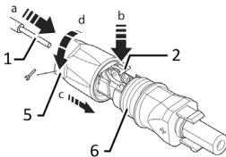
Abb. 14: Adern einfuhren
