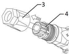
Fig. 15: Împingerea piesei detașabile în manșon
