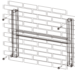
Sl. 5: Montaža zidnog držača
