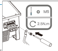
Abb. 17: Erdung anschließen
