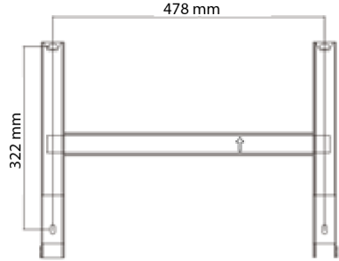
صورة رقم 4: الثقوب الخاصة بالتركيب الجداري
