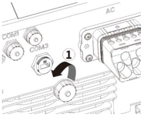
Fig. 18 : Retrait du couvercle
