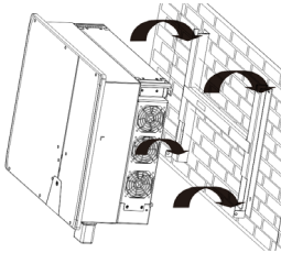
Εικ. 6: Ανάρτηση μετατροπέα στο στηρίγμα τοίχου
