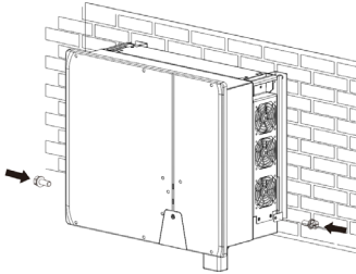
Afb. 8.1: Omvormer bevestigen
