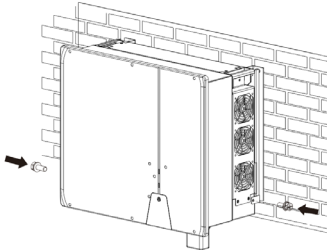
Фиг. 8.1: Закрепване на инвертор
