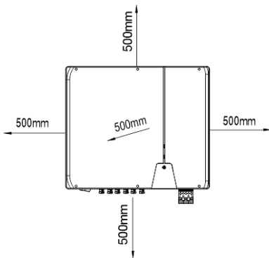
Abb. 3.1: Gerät bei Außeninstallation
