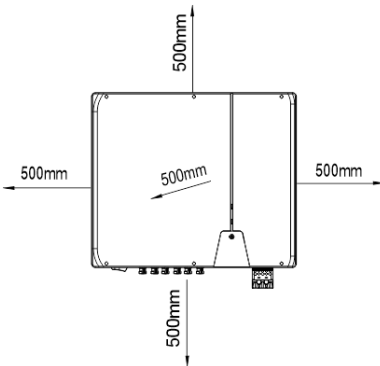
Fig. 3.1: Enhet vid installation utomhus
