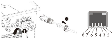
Εικ. 20: Εισαγωγή καλωδίου δικτύου
