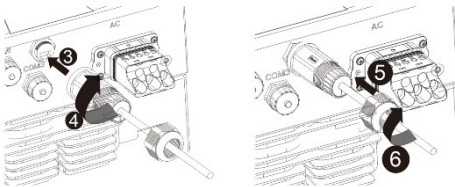
Sl. 22: Priključivanje mrežnog kabela
