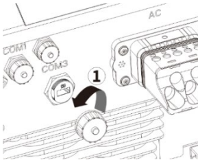
Fig. 18: Dekslret er fjernet.
