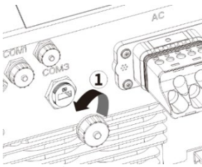
Fig. 18: Îndepărtarea apărătorii
