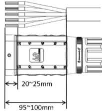
Afb. 10: Kabel voorbereiden
