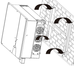
Şek. 6: İnverterin duvar tutucusuna asılması
