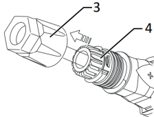
Fig. 15: Skub indsatsen ind i tyllen
