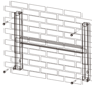
Obr. 5: Montáž nástěnného držáku
