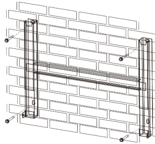
Fig. 5: Montera väggfästet
