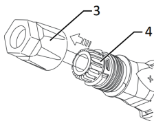
Fig. 15 : Pousser l'insert dans le manchon
