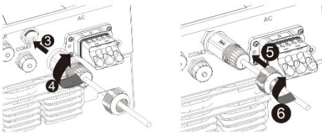
22 pav. Prijunkite tinklo kabelį
