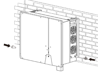
صورة رقم 1.8: تثبيت العاكس
