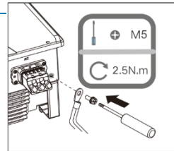
Imm. 17: Collegare la messa a terra
