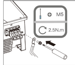
Fig. 17: Anslut till jord
