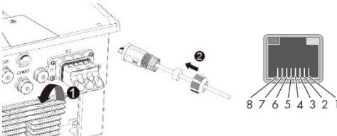
Fig. 20: Föra in nätverkskabel
