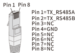
Rys. 21: Podłączenie kabla
