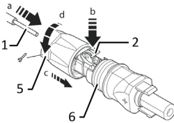
Fig. 14: Inserción de los conductores
