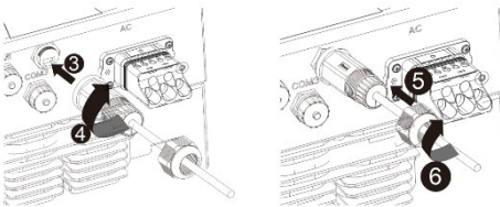
22. att. Tīkla kabeļa pieslēgšana
