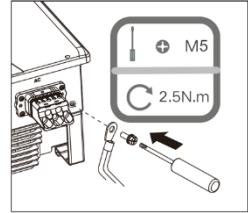
Kuva 17: Liitä maadoitus
