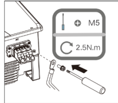
17. ábra: A földelés csatlakoztatása
