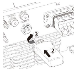
Fig. 19: Conectar el adaptador WLAN
