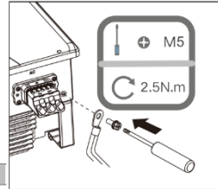
Fig. 17: Conectar la toma a tierra
