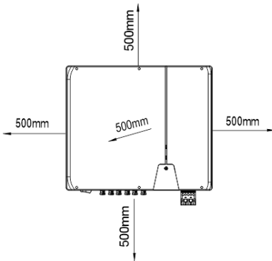
Obr. 3.1: Zařízení při venkovní instalaci
