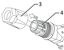
Εικ. 15: Ωθήστε το ένθεμα στην υποδοχή
