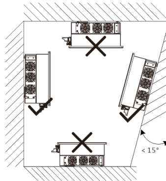
Фиг. 2: Позволено положение на разполагане
