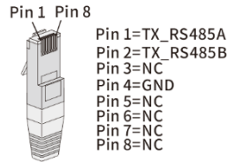
Fig. 21 : Affectation du raccord de câble
