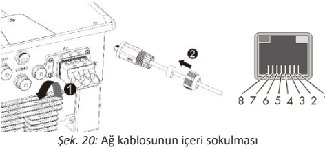
Şek. 20: Ağ kablosunun içeri sokulması
