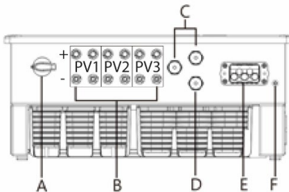
Εικ. 8.2: Πλευρά σύνδεσης: Υπόμνημα
