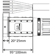
Фиг. 10: Подготовка на кабелите
