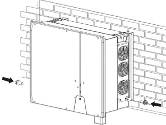
Kuva 8.1: Vaihtosuuntaimen kiinnittäminen
