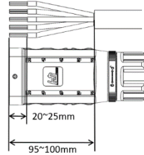
10. ábra: Kábel előkészítése
