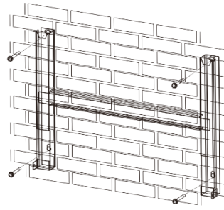
Fig. 5: Montagem do suporte de parede
