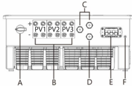
صورة رقم 8.2: جانب الوصلة: الرسوم التوضيحية
