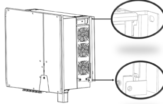
7. ábra: A készülék biztonságos illeszkedésének ellenőrzése
