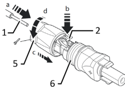
Fig. 14: Infoga ledningar
