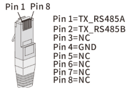
Fig. 21: Ocupação das ligações do cabo
