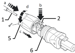
Obr. 14: Zavedení žil
