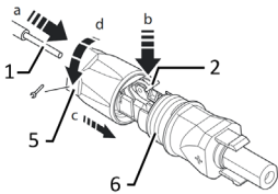
Kuva 14: Aseta johtimet paikoilleen
