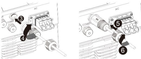
Fig. 22: Koble til nettverkskabel
