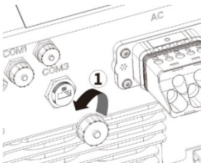
Imm. 18: Togliere la copertura
