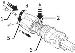
Şek. 14: Damarların içeri sokulması
