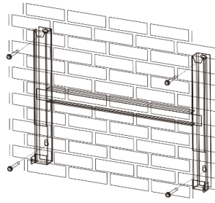
Imm. 5: Montaggio del supporto a parete
