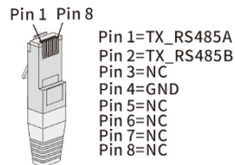
Sl. 21: Zasedenost kabljskih priključkov
