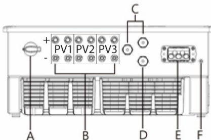
Фиг. 8.2: Страна на свързване: Легенда
