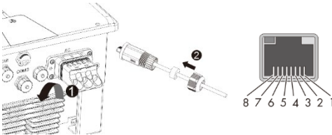
20. ábra: A hálózati kábel bevezetése
