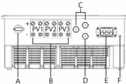
Fig. 8.2: Tilslutningsside: Tegnforklaring
