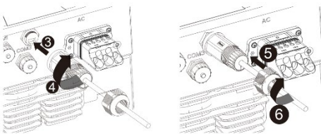
Fig. 22 : Raccordement du câble réseau
