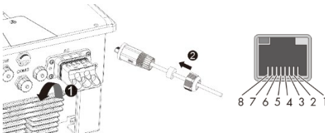
Fig. 20: Introducerea cablului de rețea
