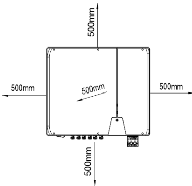
Rys. 3.1: Urządzenie przy instalacji zewnętrznej
