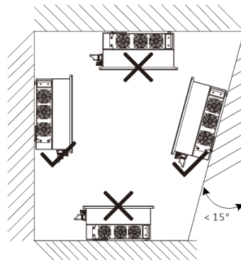
Abb. 2: Erlaubte Aufstelllage
