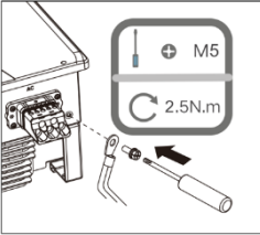
صورة رقم 17: توصيل وصلة التأريض
