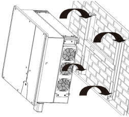
Abb. 6: Wechselrichter in die Wandhalterung einhängen
