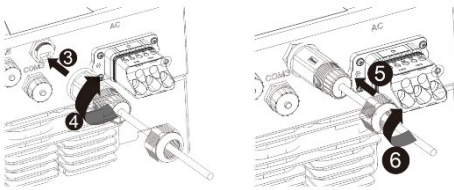
Εικ. 22: Σύνδεση καλωδίου δικτύου
