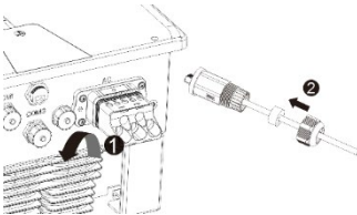
20. att. Tīkla kabeļa ievietošana
