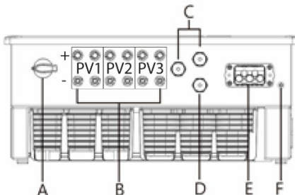
Afb. 8.2: Aansluitzijde: Legenda
