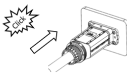
12. ábra: Burkolat behelyezése
