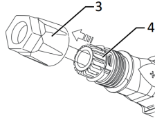
صورة رقم 15: إدخال اللقمة في الجلبة
