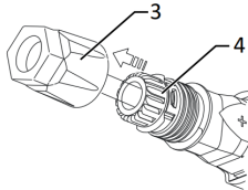
15 pav. Įstumkite įdėklą į movą
