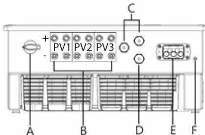
Fig. 8.2: Partea de racord: Legendă
